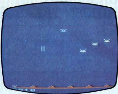
MOONBASE 10 (PDI)
