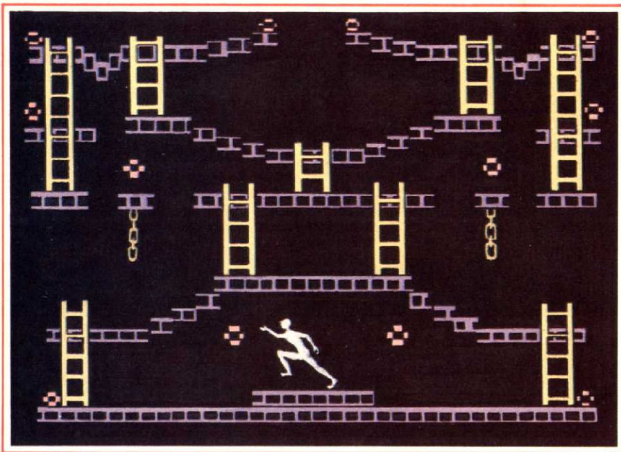
JUMPMAN
