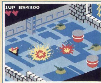
ZAXXON
