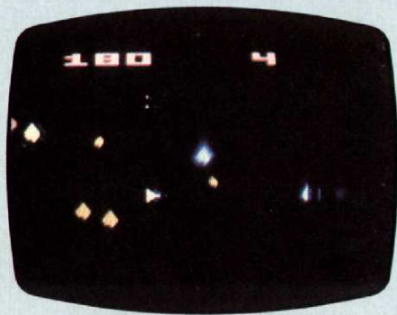
ASTEROIDS (ATARI)
