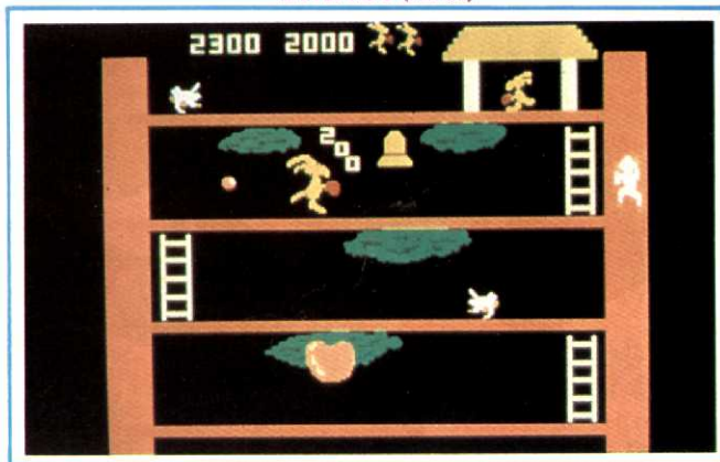
KANGAROO (ATARI)
