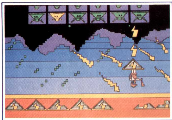
HERCULES (XONOX)
